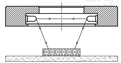
照明示意图
