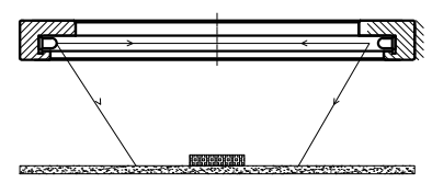
照明示意图
