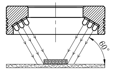
照明示意图
