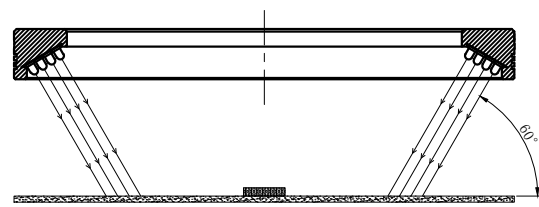
照明示意图
