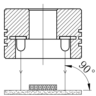
照明示意图
