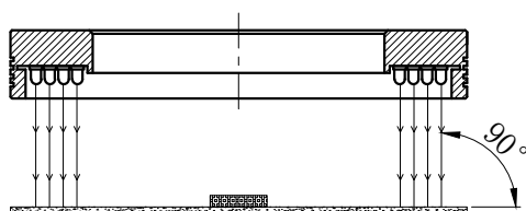
照明示意图
