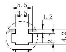
视图A, 比例2:1
