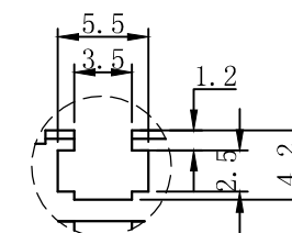
视图A, 比例2:1
