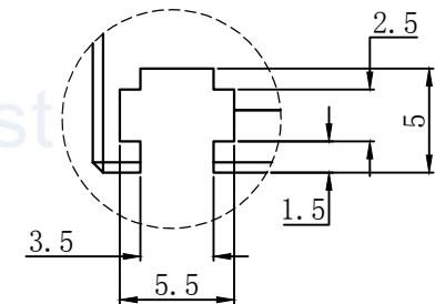
视图A 比例2:1
