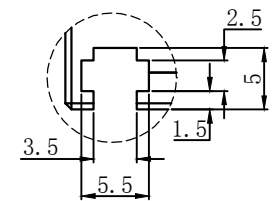
视图A 比例2:1
