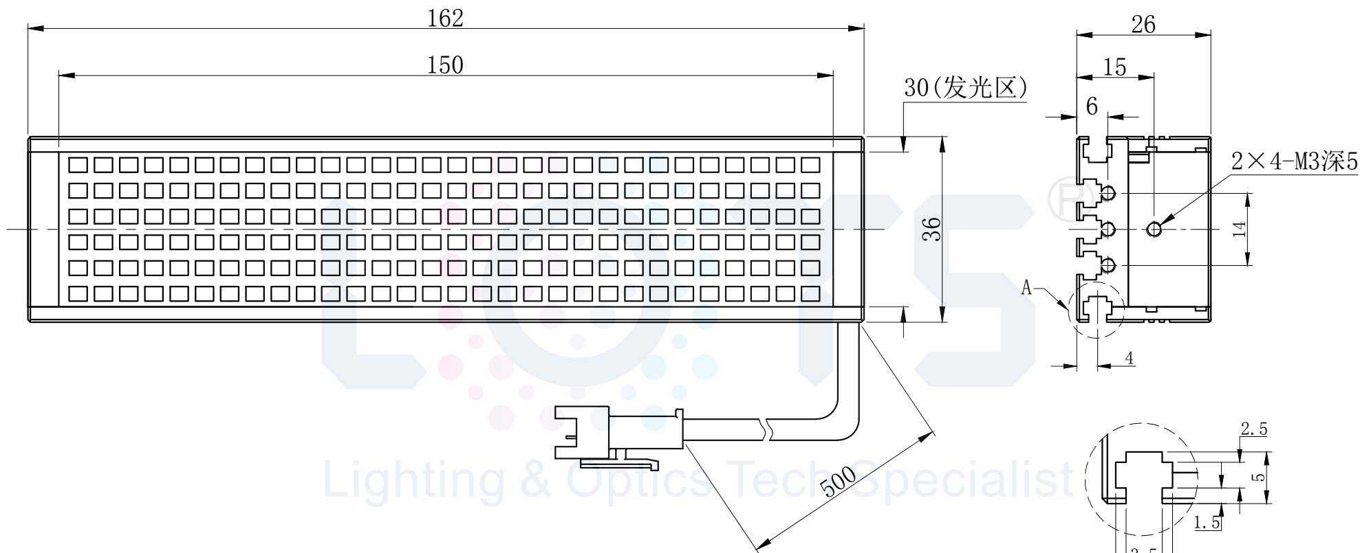
视图A 比例2: 1
