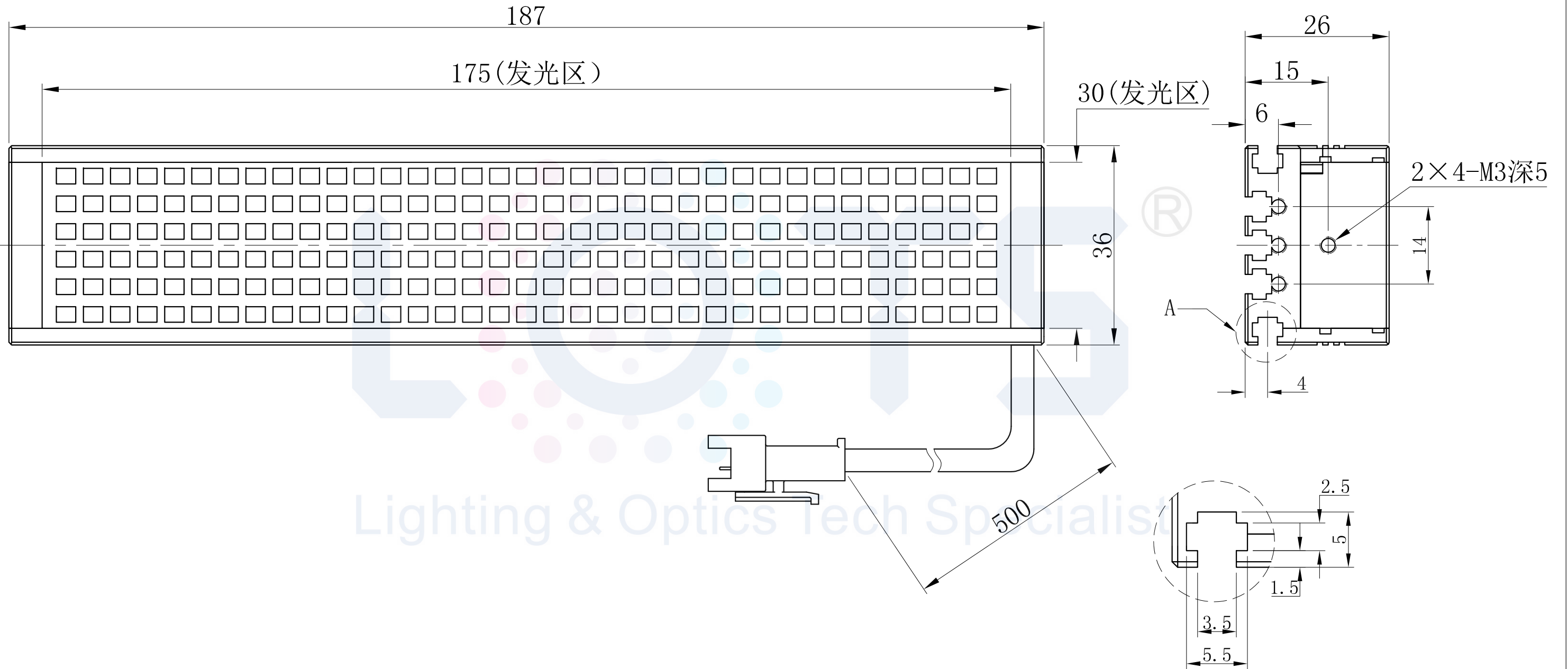
视图A 比例2: 1
