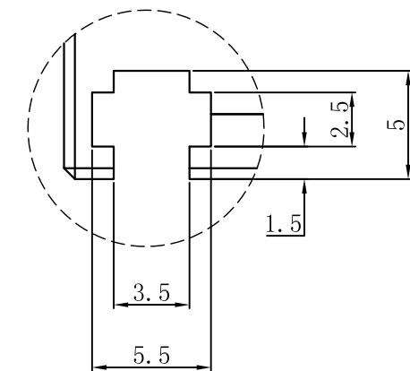
视图A 比例2: 1
