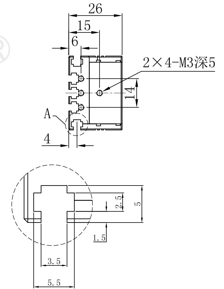
视图A 比例2: 1
