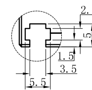
视图A 比例2:1
