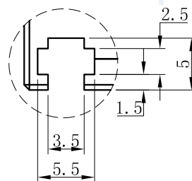
视图A 比例2:1
