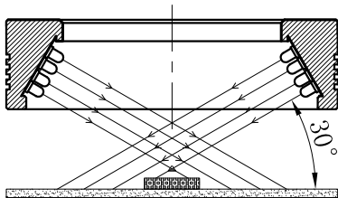
照明示意图
