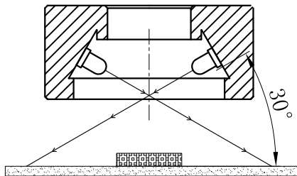
照明示意图
