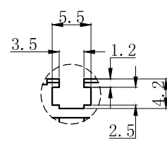
视图A, 比例2:1
