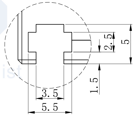
视图A 比例4: 1
