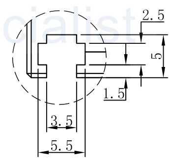
视图A 比例2: 1
