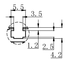
视图A, 比例2:1
