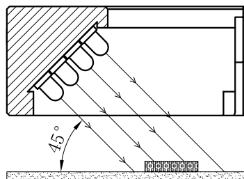
照明示意图
